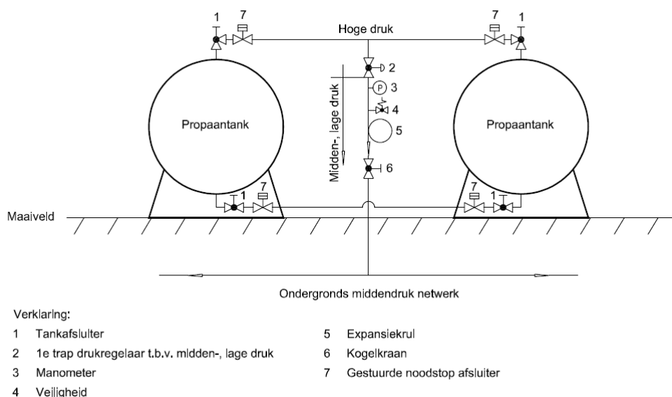
Figuur N.1 — PGS 19-opstelling met in vloeistof- en hogedrukfase gekoppelde tanks
