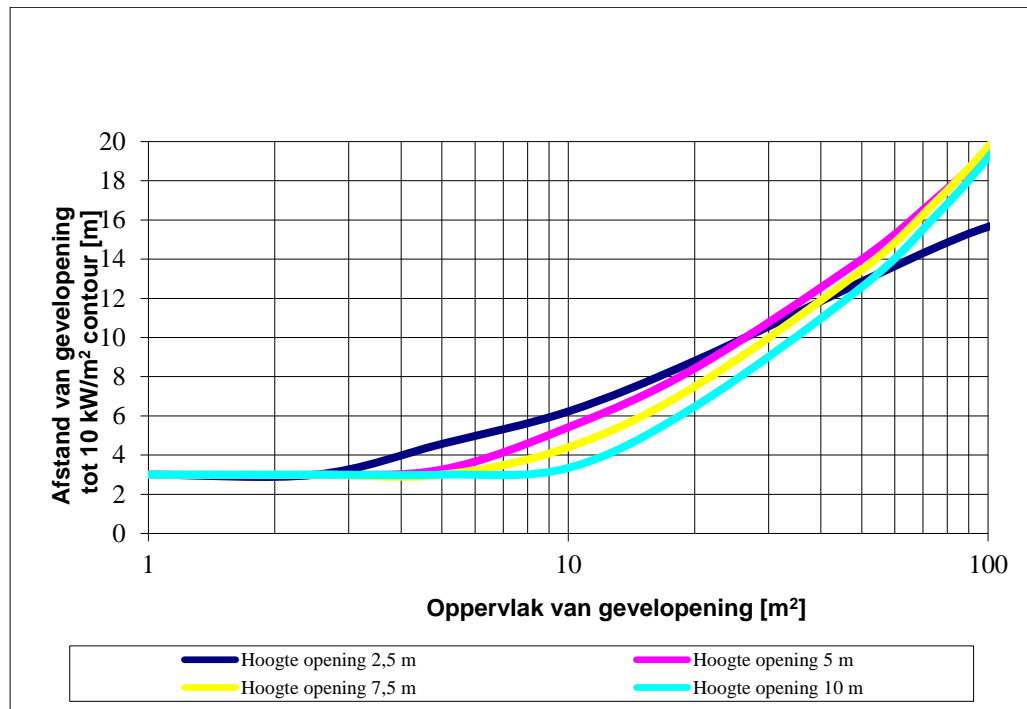
Figuur 3 — Afstand van 10 kW/m 2 -contour tot gebouwen en brandgevaarlijke opslag voor een koolwaterstofbrand
