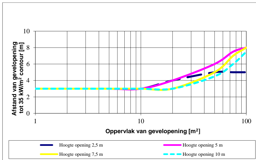
Figuur 4 — Afstand van 35 kW/m 2 -contour tot gebouwen en brandgevaarlijke opslag voor een koolwaterstofbrand
